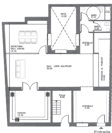
ANTEPROYECTO SEDE SOCIAL COFRADÍA LOS ESTUDIANTES
